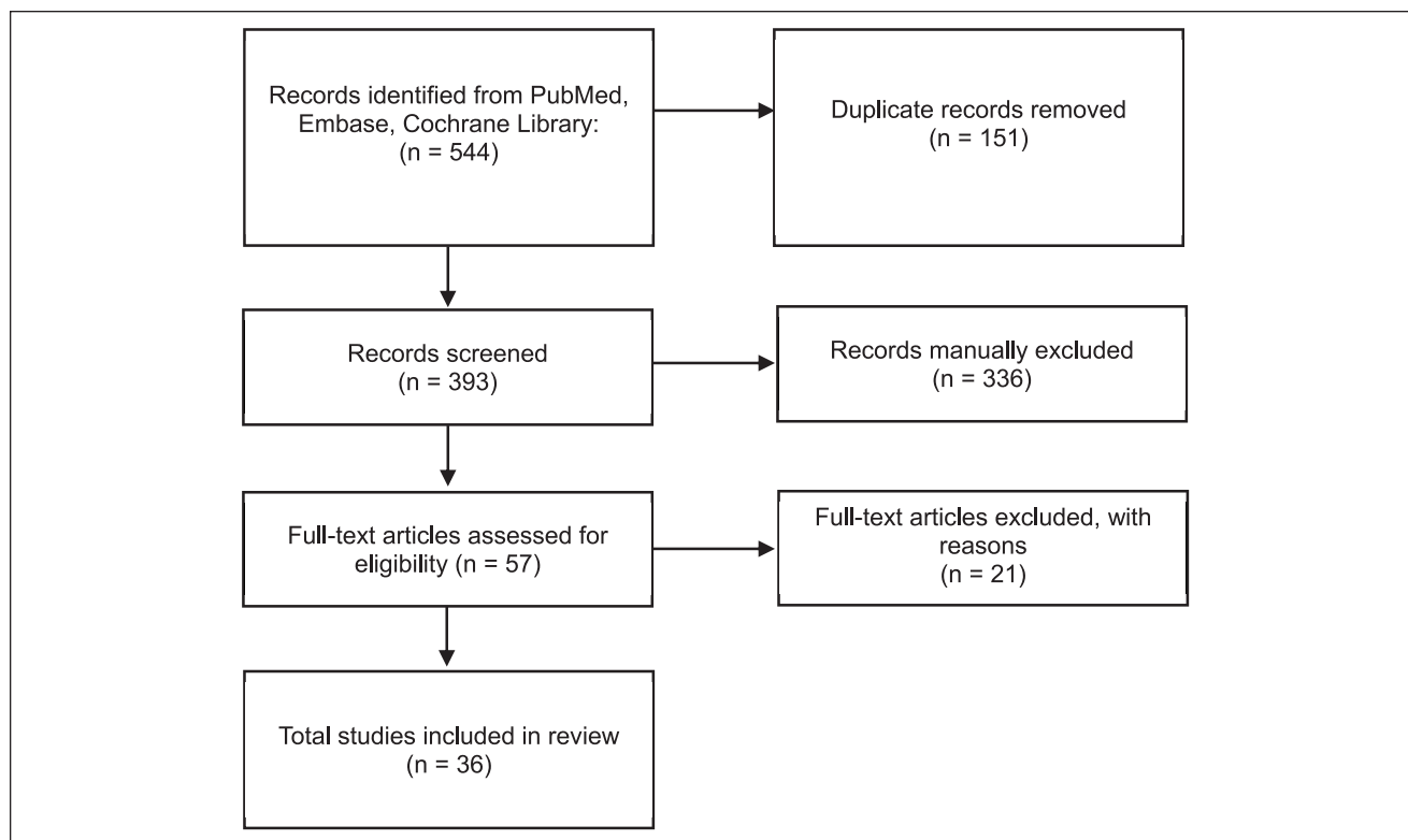
Fig. 1. PRISMA diagram.
